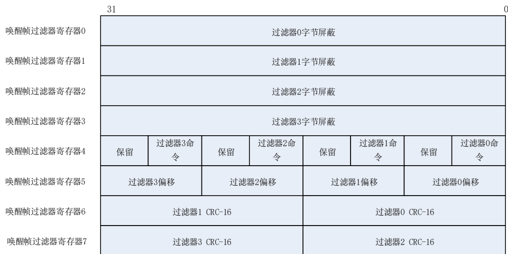
图 27-15. 远程唤醒帧过滤器寄存器
