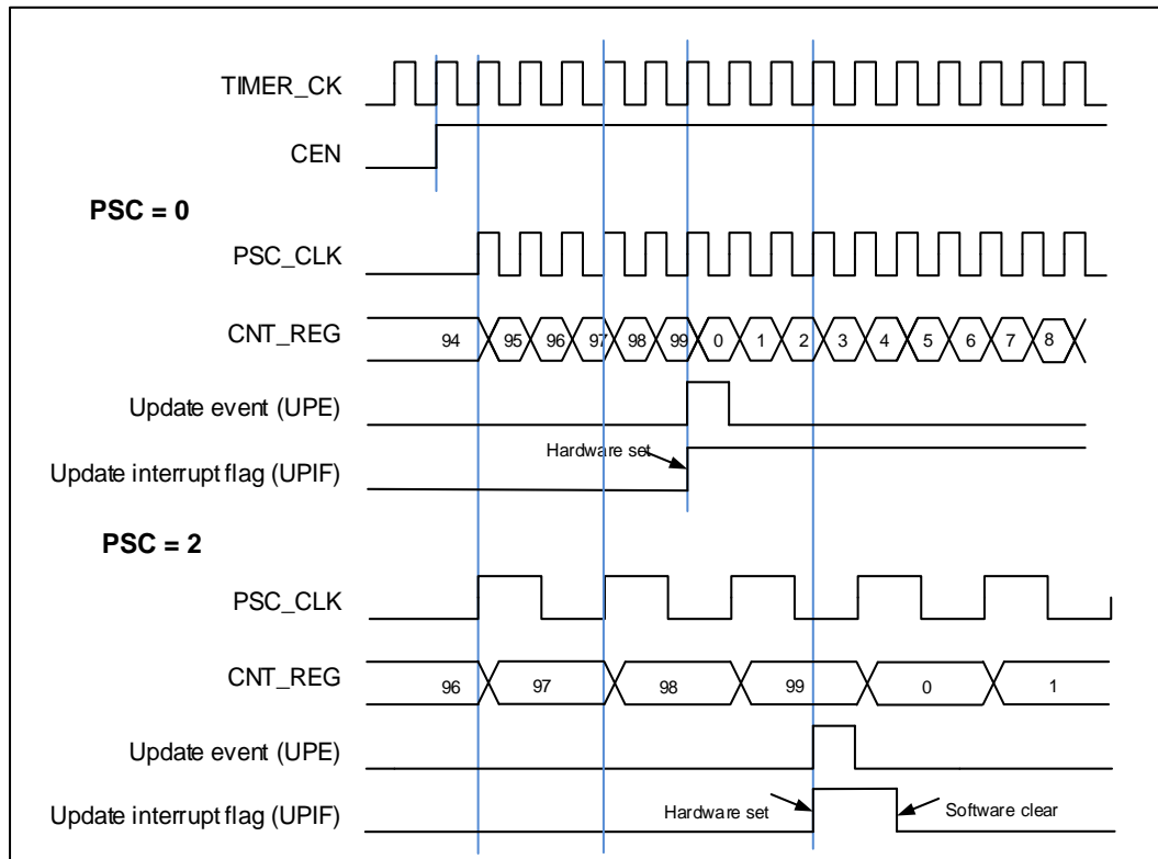
图 18-59. 向上计数时序图, PSC=0/2
