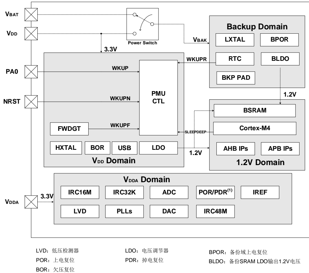
图3-1. 电源域概览
