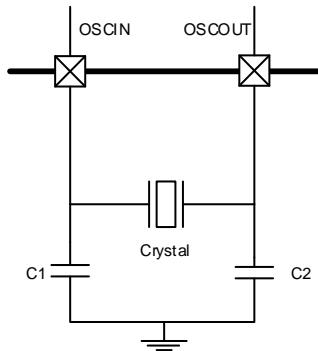
图4-3. HXTAL时钟源
