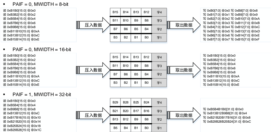
图 10-5. PWIDTH 为‘2b01’时，数据的打包/解包
