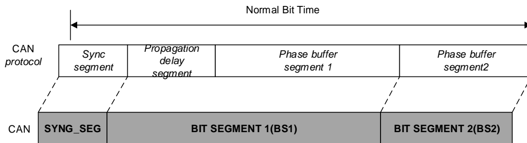
图 26-11. 位时序
