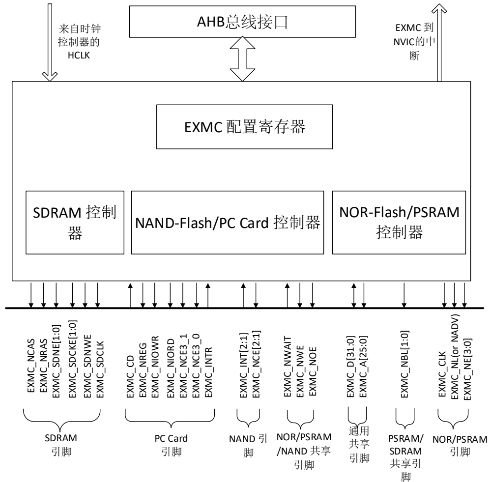
图 25-1. 系统架构
