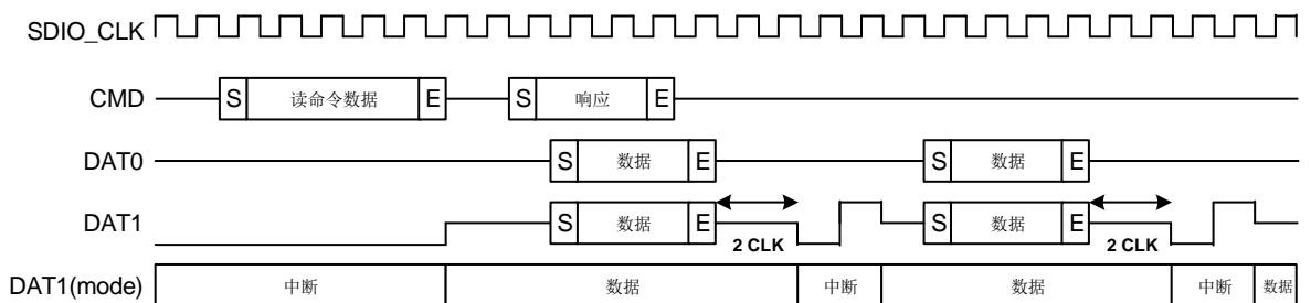
图 24-17. 4 位模式下多块读中断周期时序
