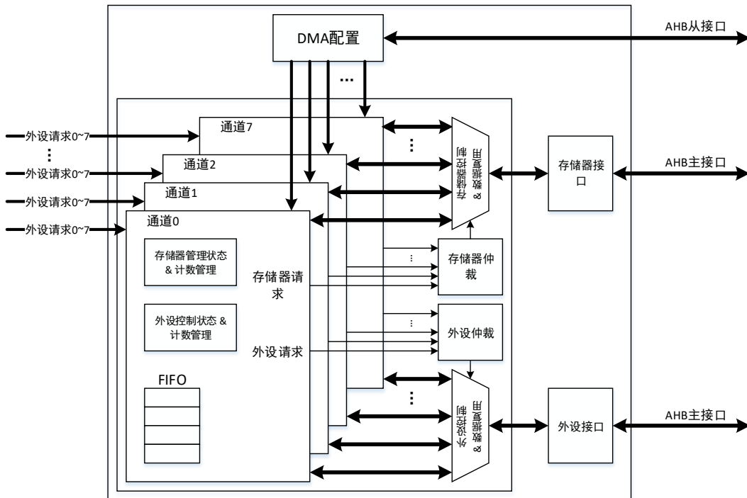
图 10-1. 系统架构
