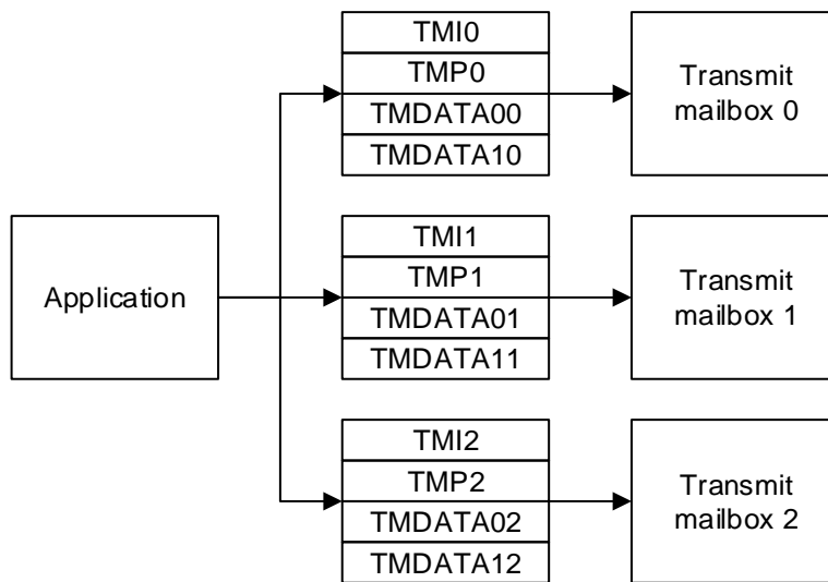
图 26-2. 发送寄存器
