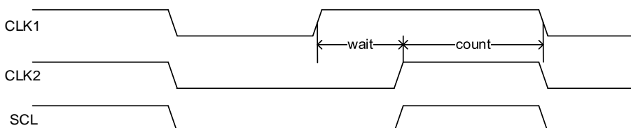
图 20-4. 时钟同步
